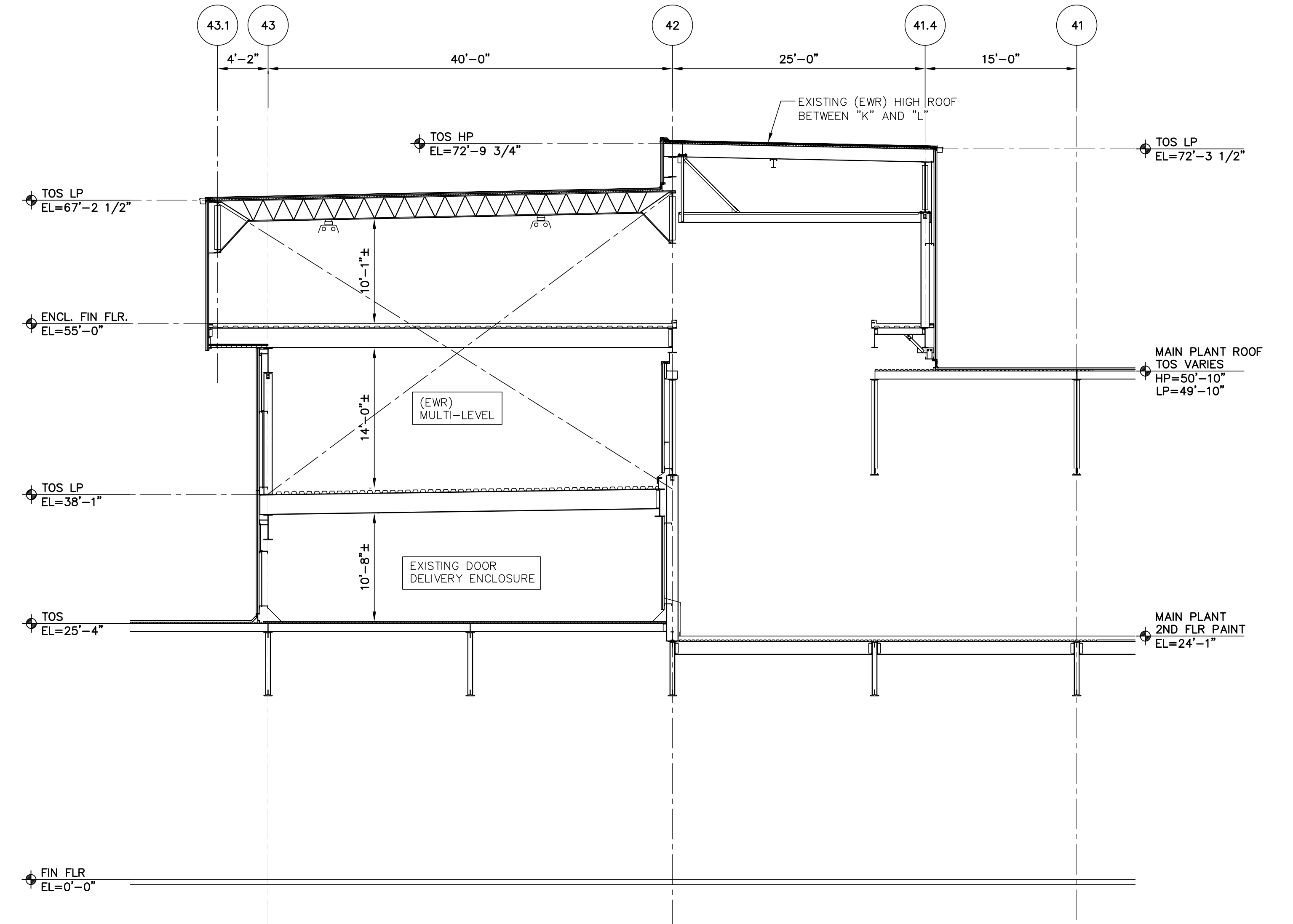
3 BUILDING SECTION A-1 SCALE: 1/8" = 1'-0"
