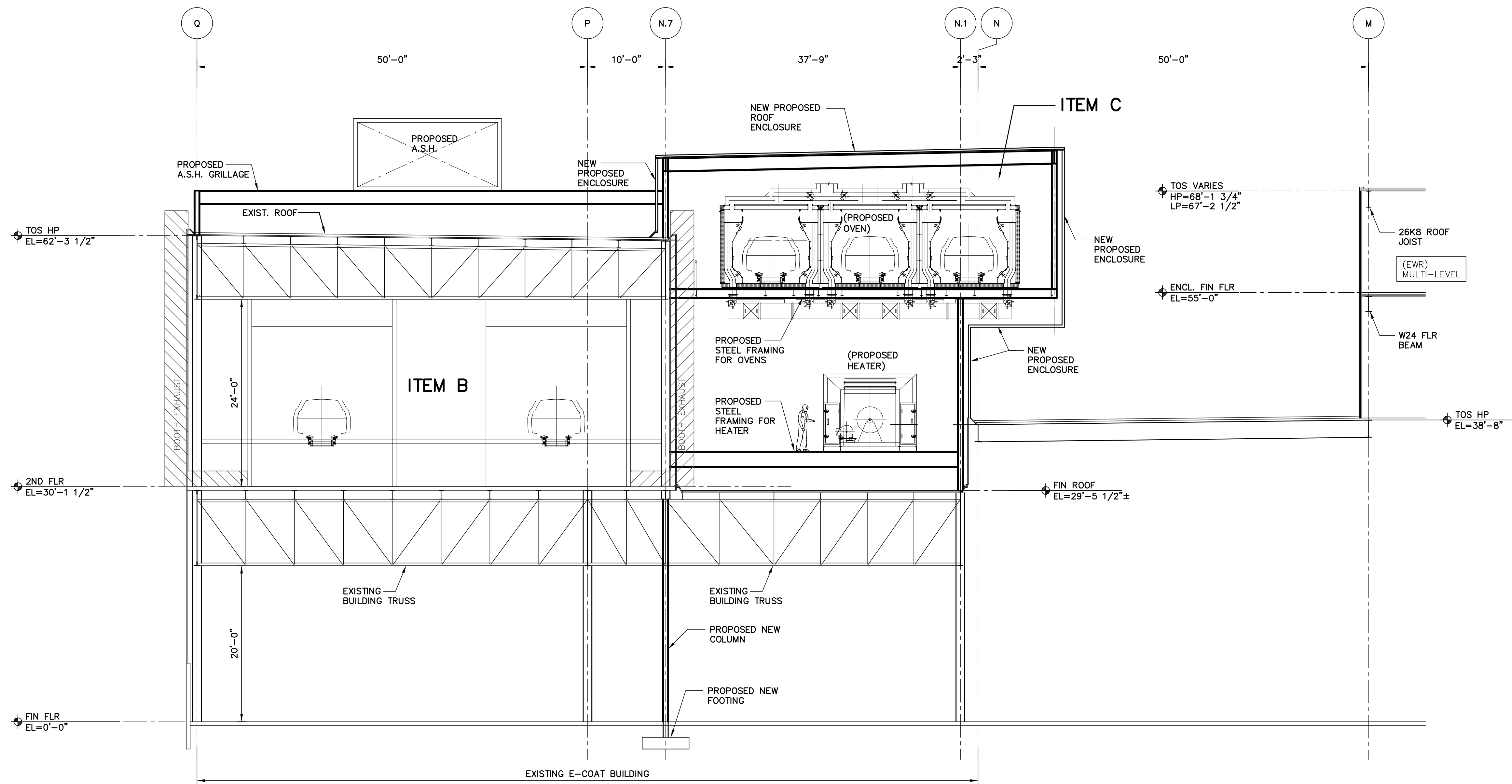
1 BUILDING SECTION A-1 SCALE: 1/8" = 1'-0"
